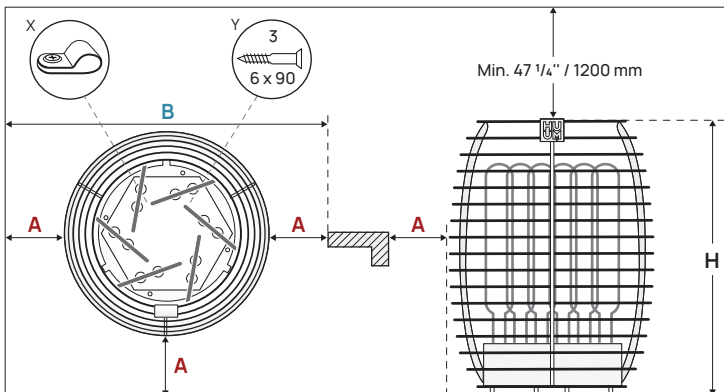
Figure 1. Positionnement du chauffe-sauna
