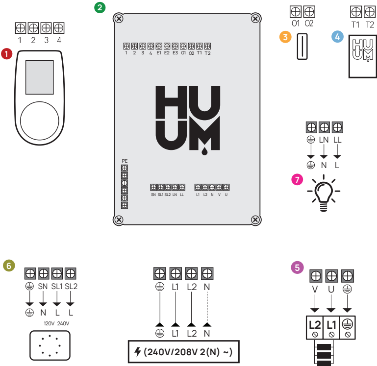
Figure 1. Connexions électriques du chauffe.
