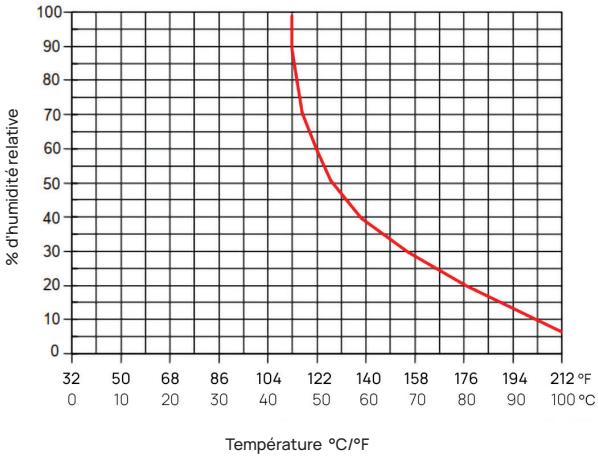
Figure 5. Caractéristiques de température et d'humidité relative en fonctionnement normal.
